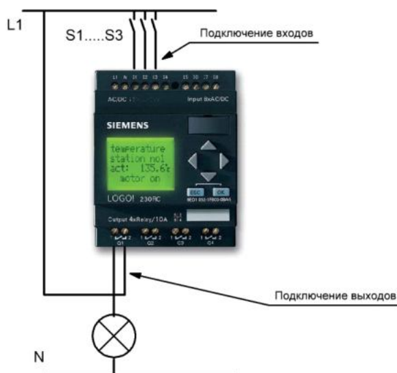
Рис.3 Монтаж Программируемого реле
