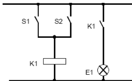
Рис.6 Коммутационная схема
